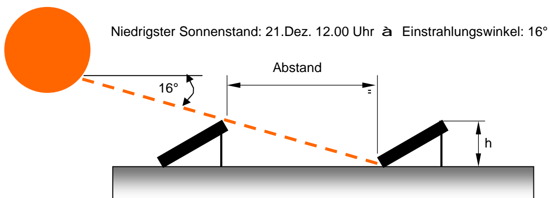
Abbildung 6-4: Abstand der Modulreihen bei Flachdachmontage
